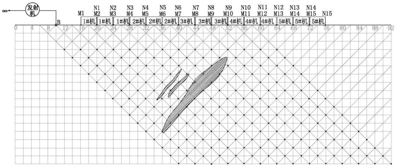
图 E.6 15 道轴向单极-偶极拟断面窗口测深布极图 ( \infty BMN 方向)
