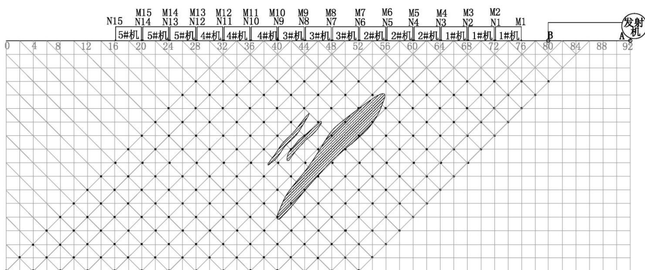
图 E.2 15 道轴向偶极-偶极拟断面窗口测深布极图 (NMBA 方向)
