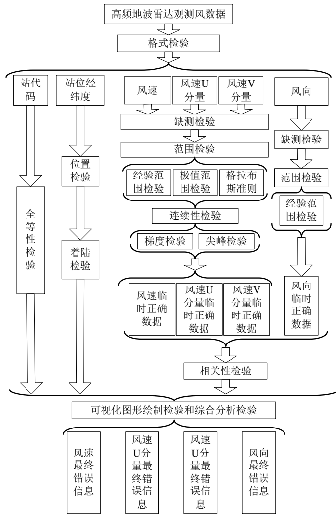
图14 高频地波雷达观测风数据质量控制流程图
