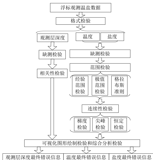
图7 浮标观测温盐数据质量控制流程图
