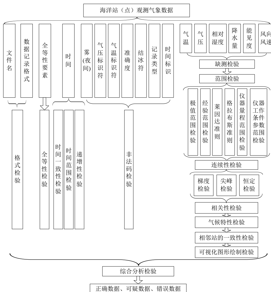
图5 海洋站(点)观测气象数据质量控制流程
