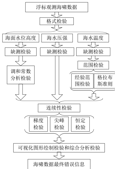
图10 浮标观测海啸数据质量控制流程
