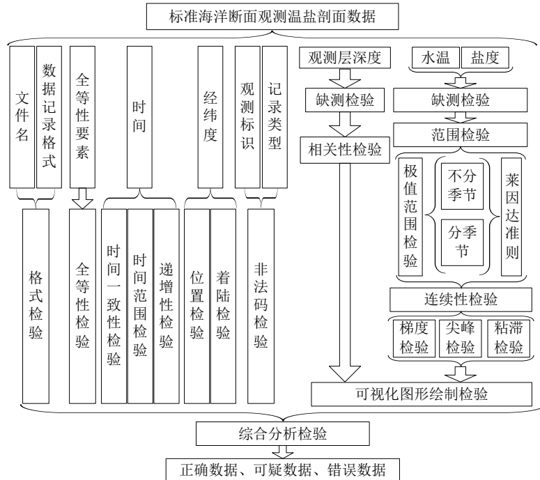
图15 标准海洋断面观测温盐剖面数据质量控制流程图
