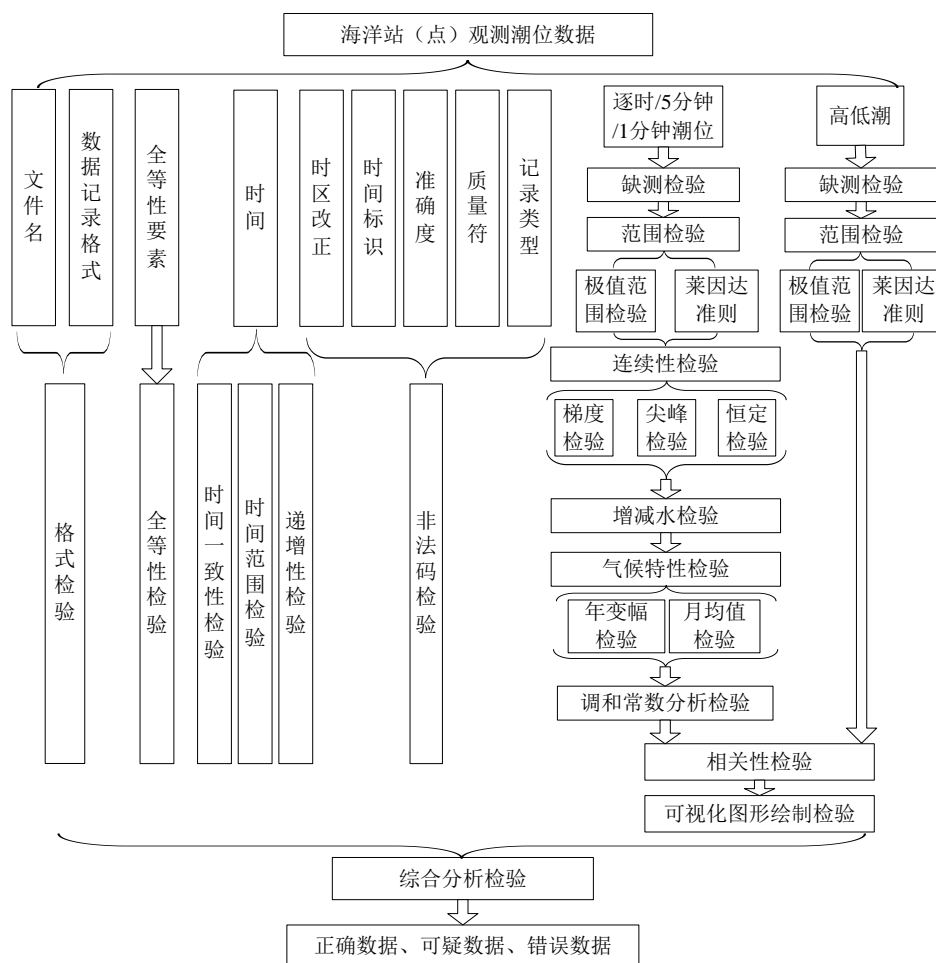
图2 海洋站(点)观测潮位数据质量控制流程
