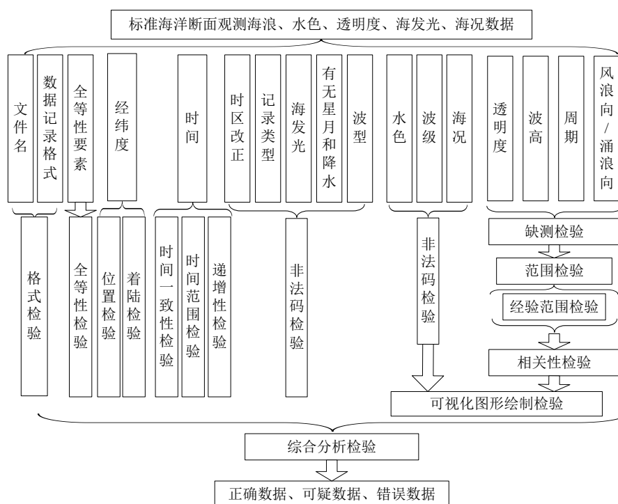
图17 标准海洋断面观测海浪、水色、透明度、海发光、海况观测数据质量控制流程图
