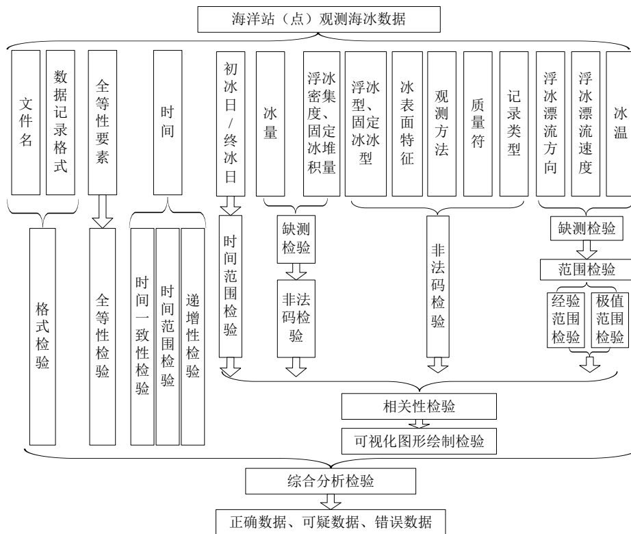
图4 海洋站(点)观测海冰数据质量控制流程
