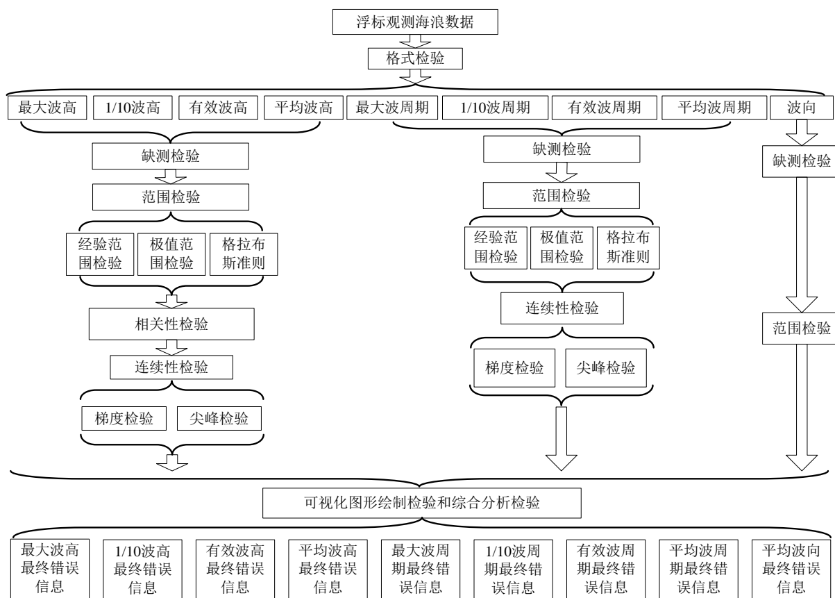
图8 浮标观测海浪数据质量控制流程图
