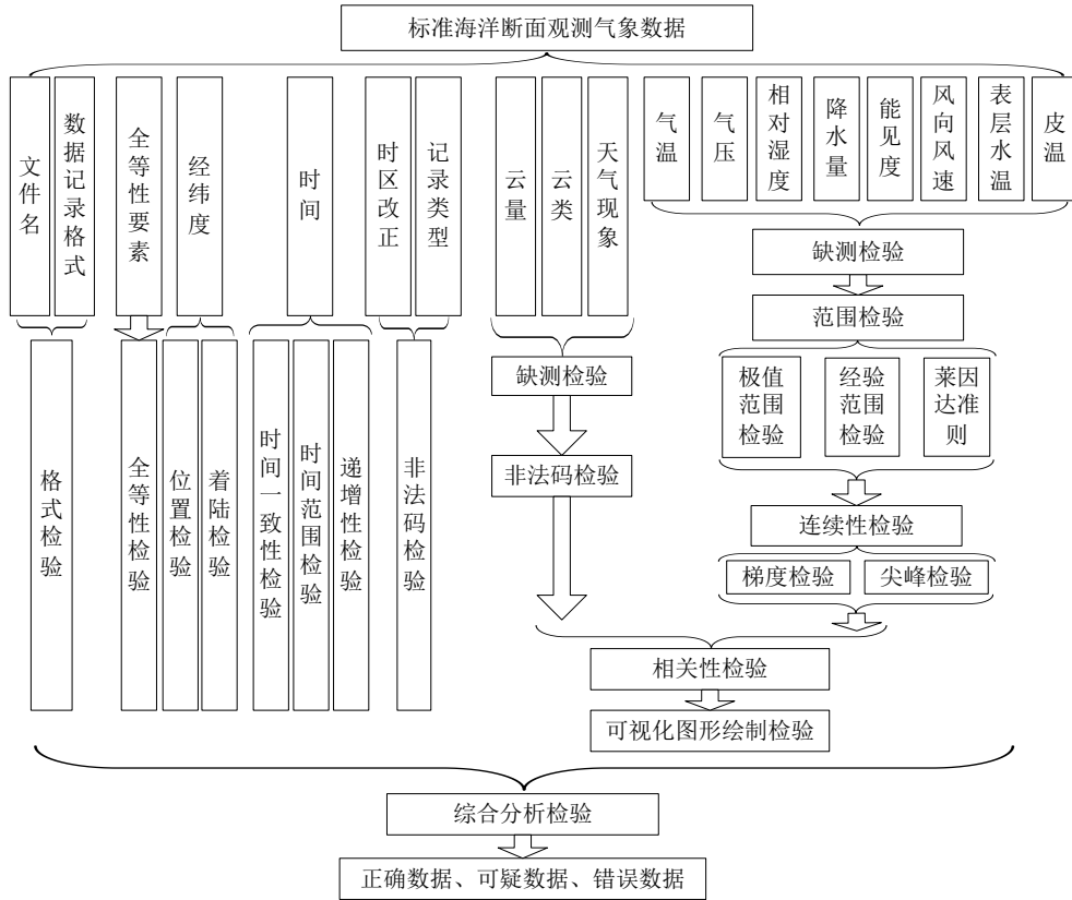
图16 标准海洋断面观测气象数据质量控制流程图
