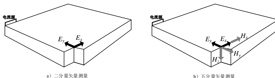
图A.5 矢量测量方式
