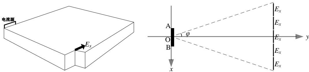
图A.1 E-E_x 旁侧装置测量形式
