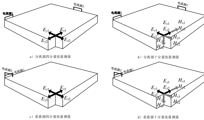
图A.6 张量测量方式
