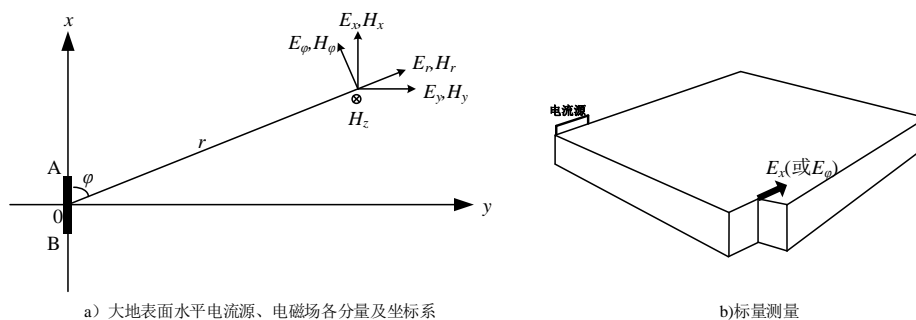
图A.4 标量测量方式
