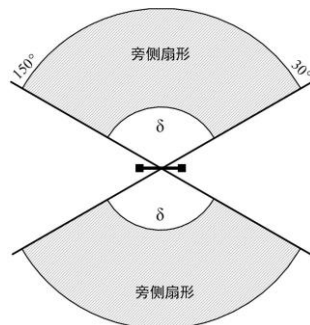
图A.8 E-E_\phi 装置的测量范围示意图
