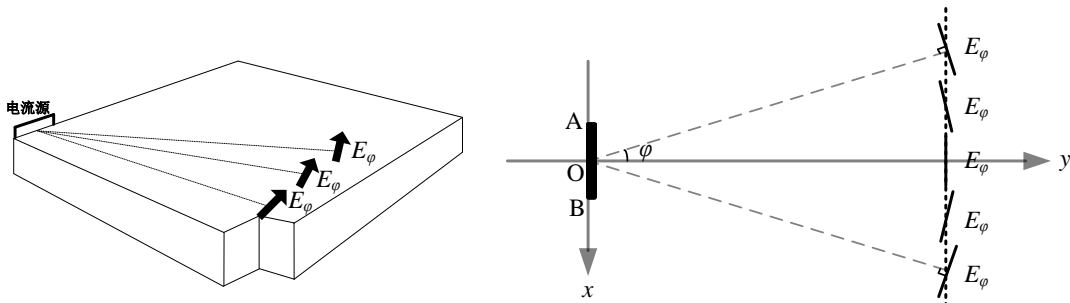
图A.3 E-E_\phi 装置测量形式
