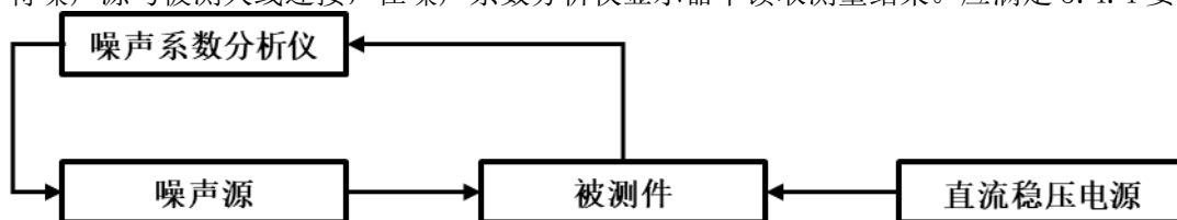
图2 LNA 噪声系数测量框图
