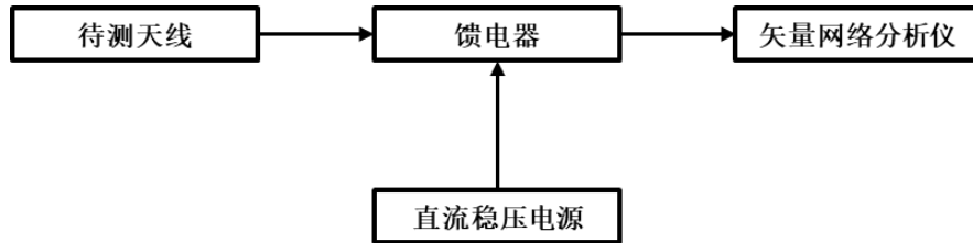
图1 网络分析仪法测量有源天线 VSWR 的框图
