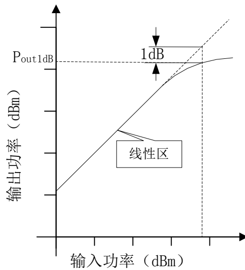
图5 输出功率与输入功率响应曲线图
