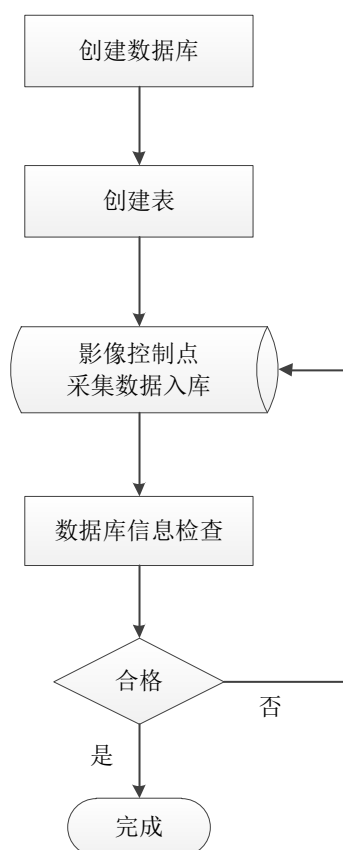
图2 影像控制点采集数据入库流程
