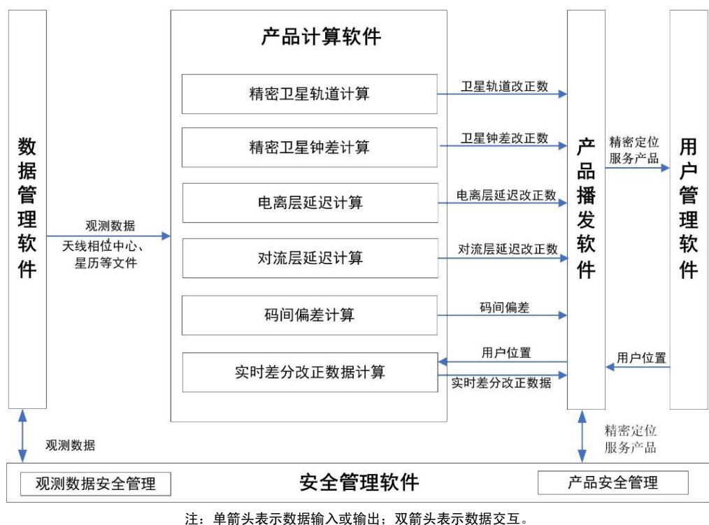
图 2 数据中心软件组成
